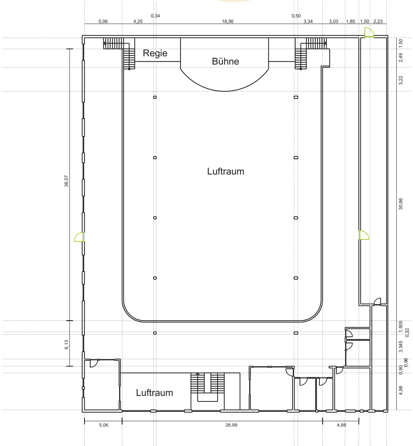
Grundriss Empore Maßstab 1:300
